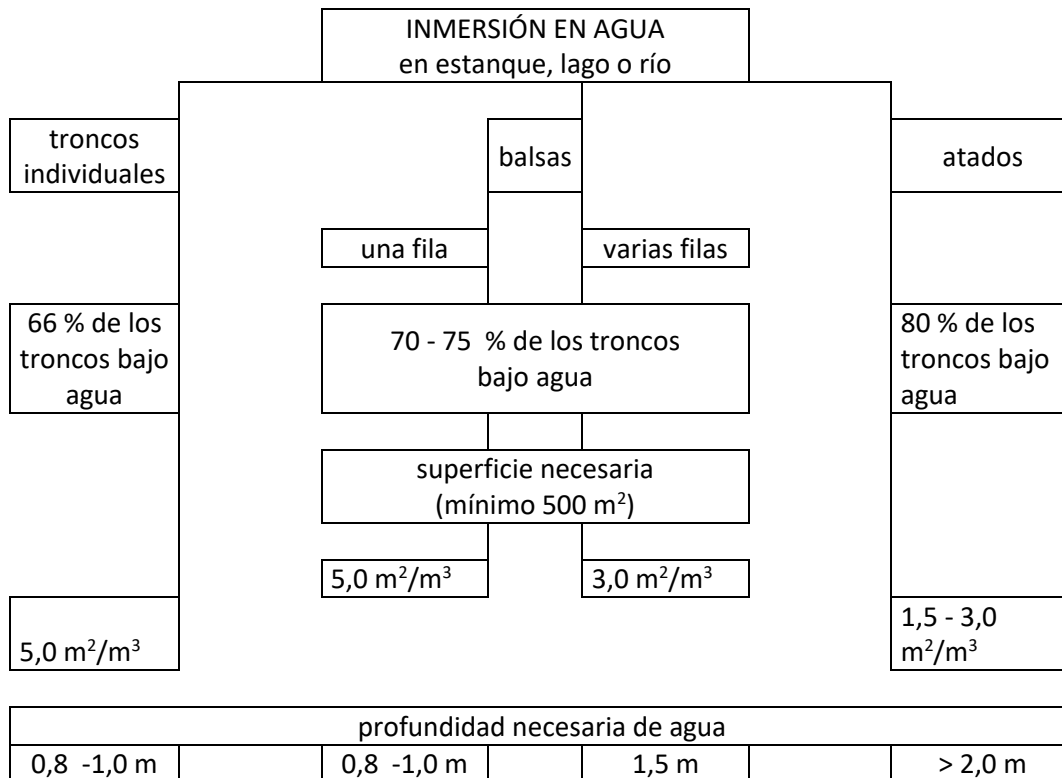
Fig. 3 Requisitos de superficie y profundidad para diferentes sistemas de inmersión de troncos. Este esquema se basa en corrientes de agua (Patzak & Löffler, 1988)
